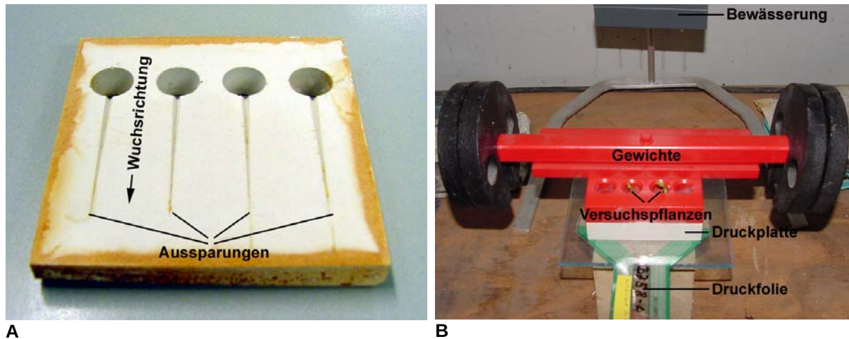
Abb. 15: Versuchsaufbau für Druckmessungen an Wurzeln. A Druckplatte aus Gips. Die braune Färbung wird durch Oxidation der Gussform ausgelöst, die als äußere Begrenzung bei Herstellung der Platten eingesetzt wurde. Sie hat keine Auswirkungen auf den Verlauf der Versuche. B Versuchsaufbau zur Messung des Wurzeldruckes. Es sind zwei Versuchspflanzen erkennbar.
