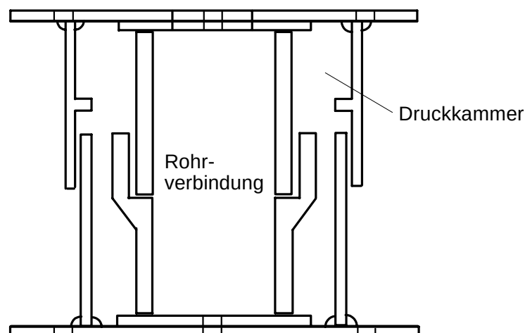
Abb. 22 : Entwurf eines Außendichtheitsprüfgerätes.
