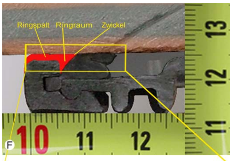
Abb. 18: Bestimmung der Dichmittelgeometrie durch optischen Vergleich [mm].
