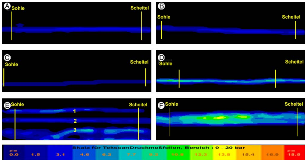
Abb. 20: Anpressdruckverteilung unterschiedlicher Rohrverbindungen ohne Scherlast. A Eurotop-Verbindung, Versuch ohne Scherwegbegrenzung. B Eurotop-Verbindung, Versuch mit Scherwegbegrenzung. C Eurotrad-Verbindung. D Cerafix-Verbindung. E KG-Rohrverbindung (PVC-U). F Tyton-Verbindung.
