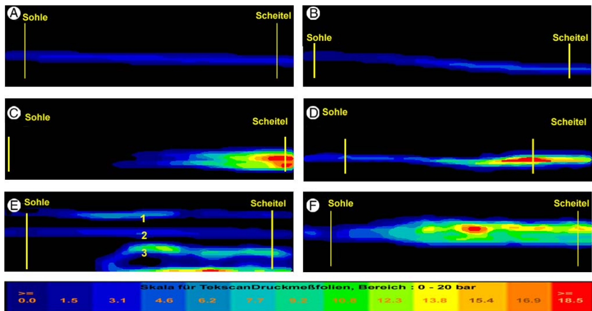
Abb. 21: Anpressdruckverteilung unterschiedlicher Rohrverbindungen unter maximaler Scherlast. A Eurotop-Verbindung ohne Schwerwegbegrenzung. F_s = 3750 N B Eurotop-Verbindung mit Schwerwegbegrenzung. F_s = 3750 N C Eurotrad-Verbindung. F_s = 3750 N D Cerafix-Verbindung. F_s = 3750 N E KG-Rohrverbindung (PVC-U). F_s = 1539 N F Tyton-Verbindung. F_s = 4500 N.
