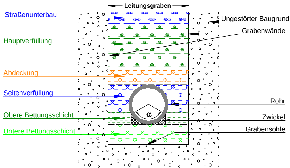
Abb. 3: Baugrundzonen nach DIN EN 1610 [10].
