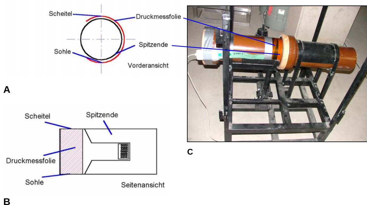
Abb. 19: Messung des Anpressdruckes bei Einwirken einer Scherlast. A Druckfolie auf dem Spitzende einer Rohrverbindung, Querschnitt. B Druckfolie auf dem Spitzende einer Rohrverbindung, Ansicht. C In den Scherlastversuchsstand eingebaute Rohrverbindung.
