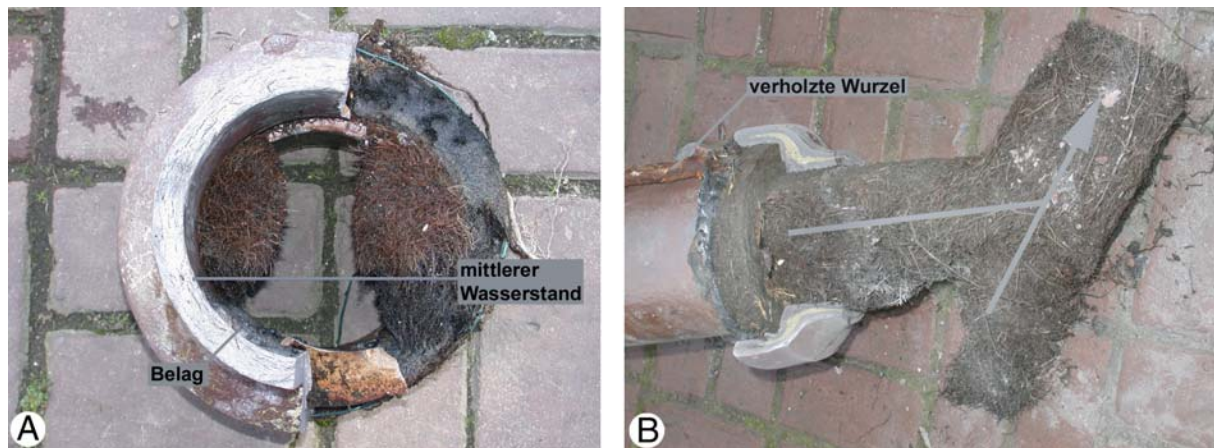
Abb. 5 Die Ausbreitung von Wurzeln in einer Leitung variiert mit der Art des Leitungsmediums. A In Mischwasser- bzw. Schmutzwasserleitungen wachsen Wurzelpolster hauptsächlich in Bereichen, die nicht oder nur selten mit Abwasser in Kontakt kommen (oberhalb des mittleren Wasserstandes). B In Regenwasserleitungen breiten sich die Wurzeln auch in wasserführenden Bereichen (Sohle der Leitung) aus.
